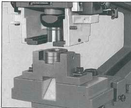
Stanzausrüstung zur Aufnahme von Stempel und Matrizen von 30,5 bis 50 mm Schnitt- \emptyset
