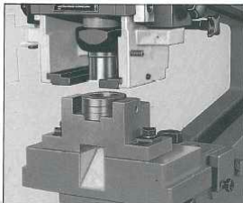
Stanzausrüstung zur Aufnahme von Stempel und Matrizen von 30,5 bis 50 mm Schnitt-Ø
