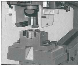
Stanzausrüstung zur Aufnahme von Stempel und Matrizen von 30,5 bis 50 mm Schnitt- \phi
