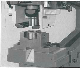
Stanzausrüstung zur Aufnahme von Stempel und Matrizen von 30,5 bis 50 mm Schnitt- \phi
